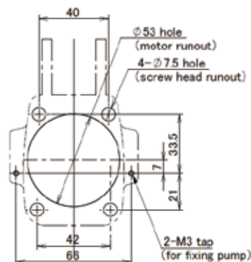
【Mounting plate view】
