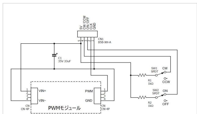
〔制御基板の接続回路例〕
