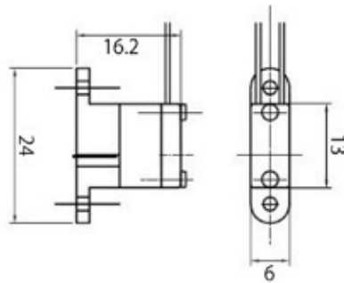
外観寸法図
